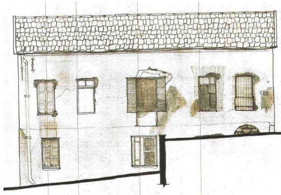
חזית מבנה לרוחב בנימין מ.ד. אשכנזי אדריכלים, תיק תיעוד
