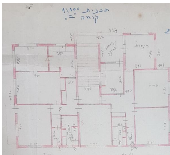
תכנית קומה ב' של בית המלון
